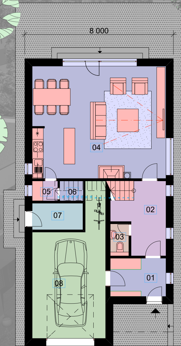
PŮDORYS 1.NP
